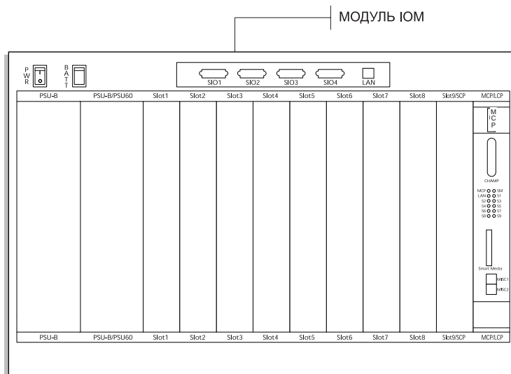
Рис. 3-16 Нумерация и название слотов
