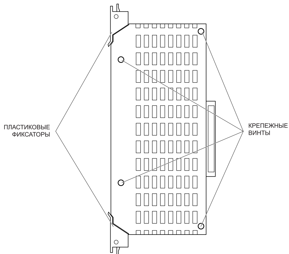
Рис. 3-19 Снятие корпуса с карты TEPR1
