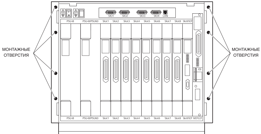
Рис.2-5 Установка блока в 19-тидюймовую стойку
