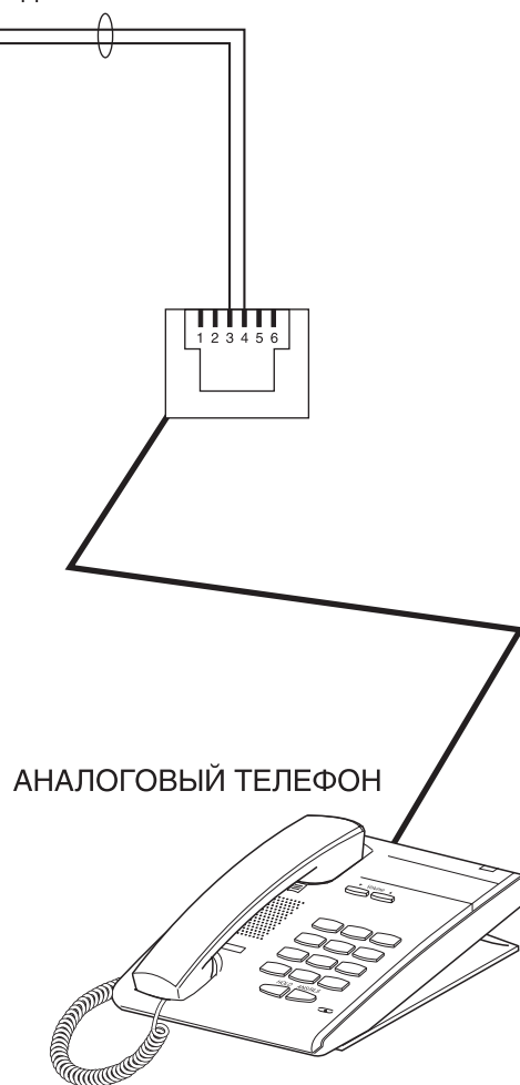
Рис. 6-2 Подключение аналоговых телефонов
