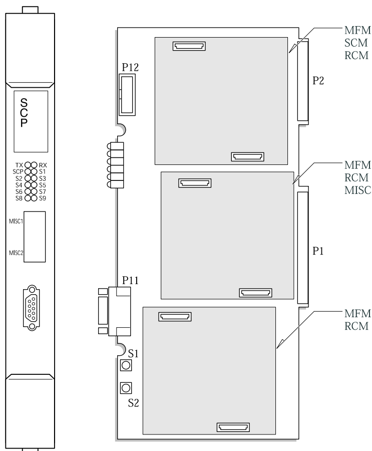
Рис. 3-3 Карта сопроцессора SCP
