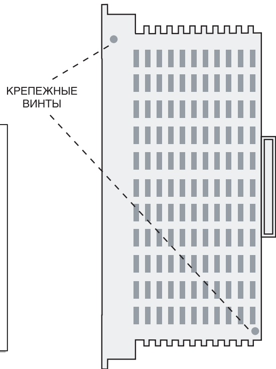
Рис. 3-6 Расположение крепежных винтов карт MCP и LCP
