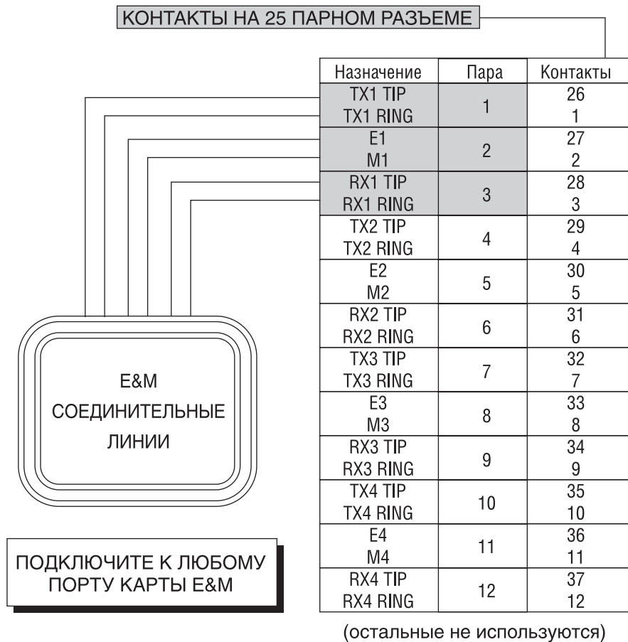
Рис. 5-3 Подключение соединительных линий E&M
