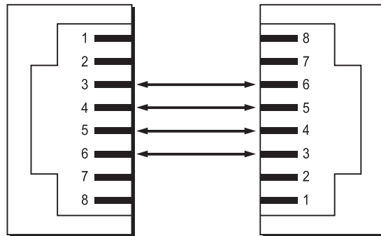
РОЗЕТКА RJ-45 ОТ 8BSI
