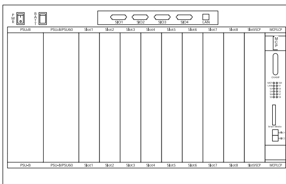
Рис. 3-2 Расположение процессора MCP
